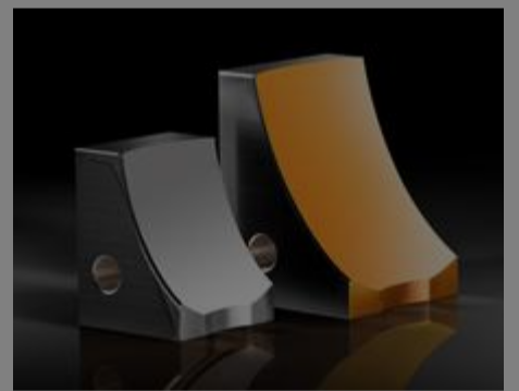
Off-Axis-Ellipsoidspiegel
