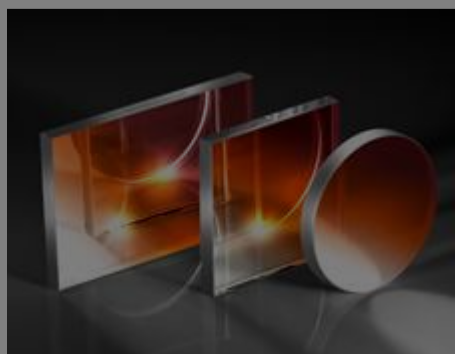
#48-901 – Strahlteilerplatte für NIR, 75 x 75 mm, 30R/70T
