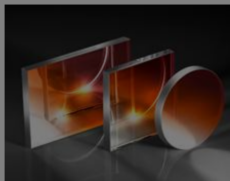
#48-904 – Strahlteilerplatte für VIS, 75 x 75 mm, 50R/50T
