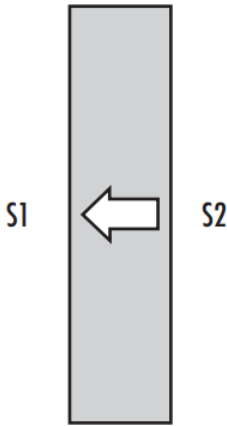
Alle gefassten optischen TECHSPEC Filter haben einen Pfeil auf dem Rand der Fassung, der auf die Seite mit der Filterbeschichtung (S1) zeigt. Die Antireflexionsbeschichtung ist auf der Seite S2 aufgebracht.
