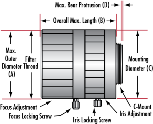
Objektiv mit Festbrennweite der C-Serie - Technische Abbildung
