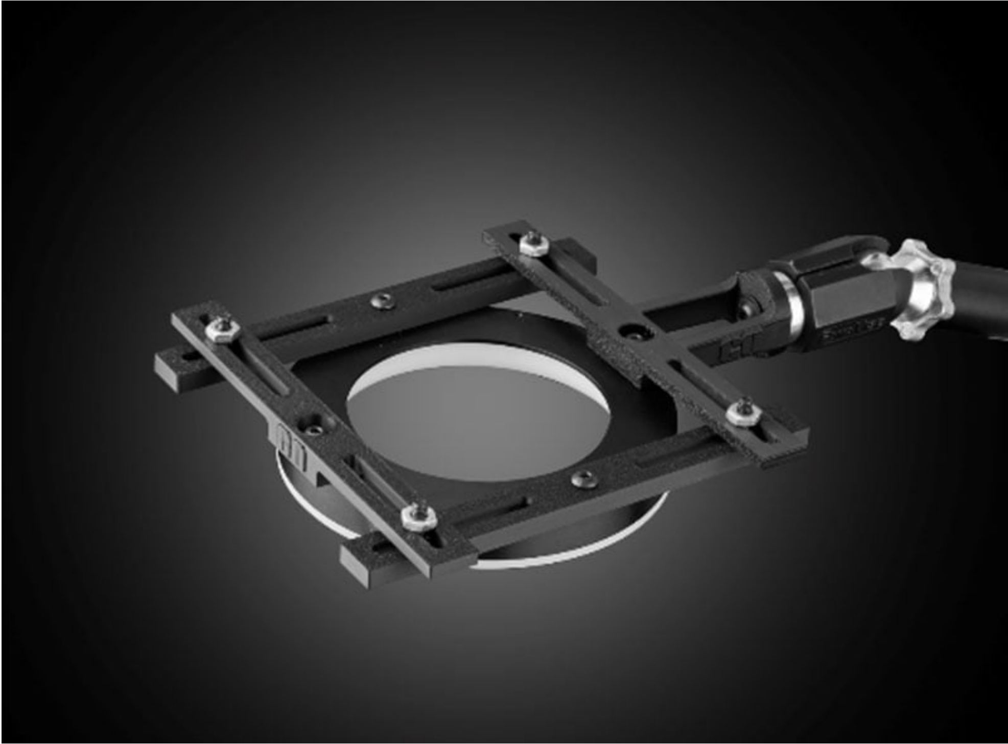
Ringlicht-Konfiguration
