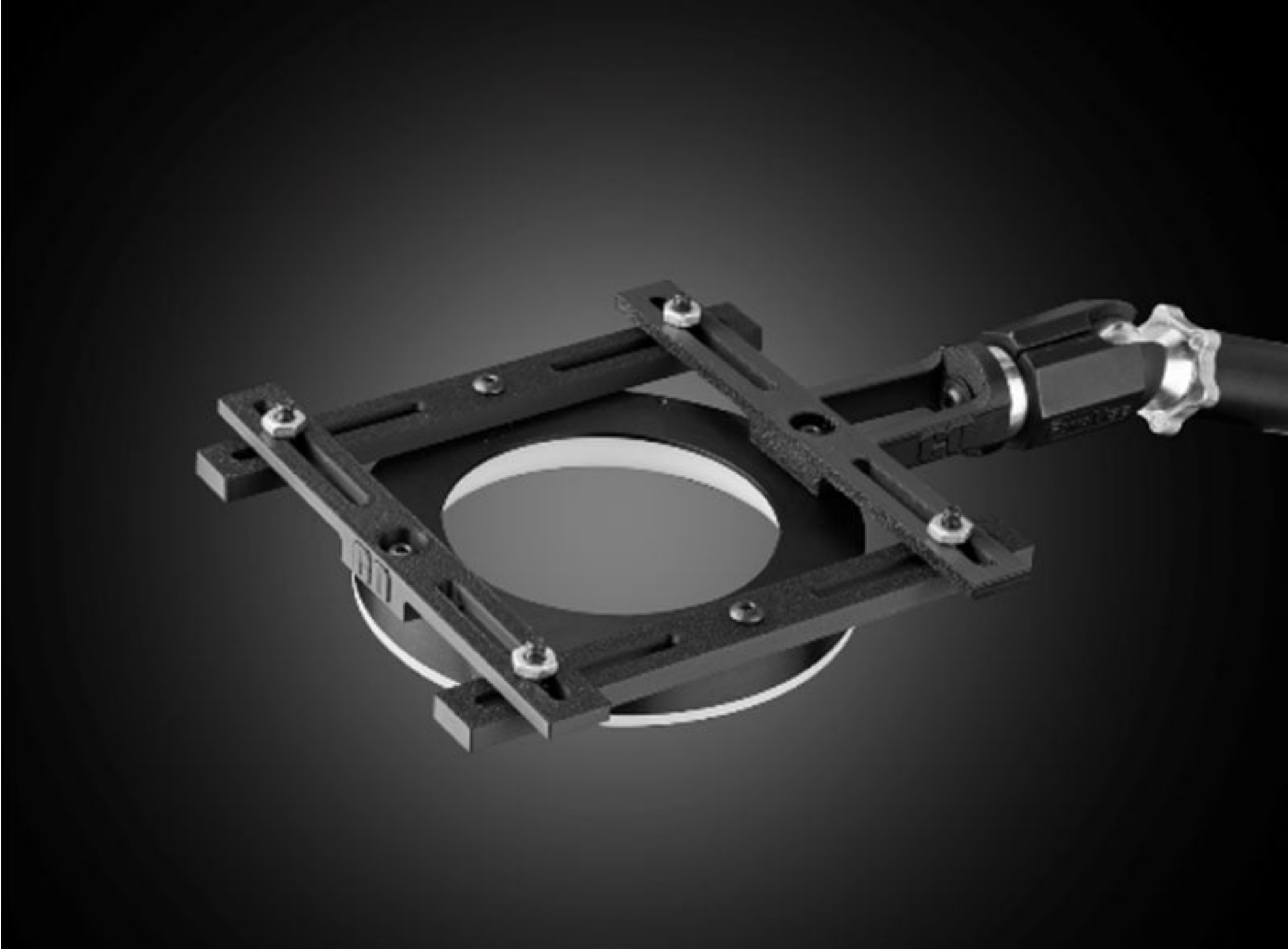
Ringlicht-Konfiguration
